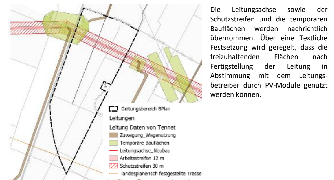
Abb. 10 Leitungsvorhaben 380-kV Conneforde-Sottrum
